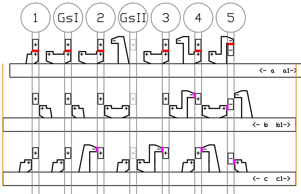
Fahrstraße a1 eingestellt
