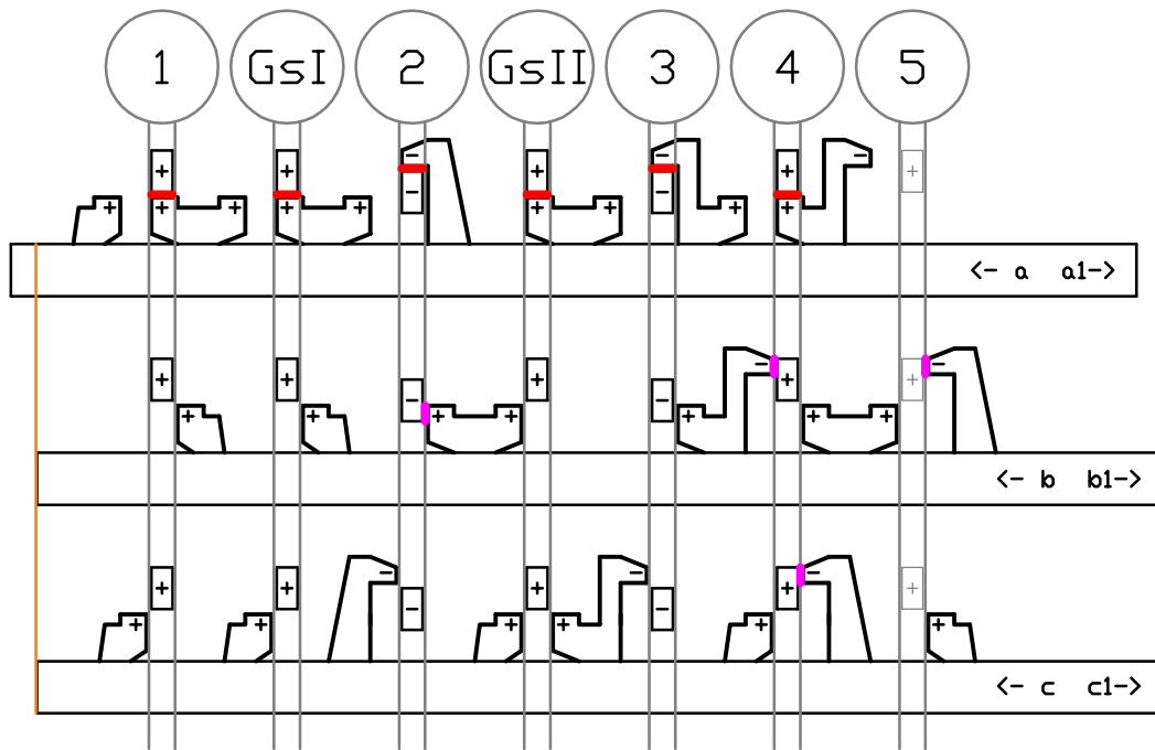
Fahrstraße a eingestellt
