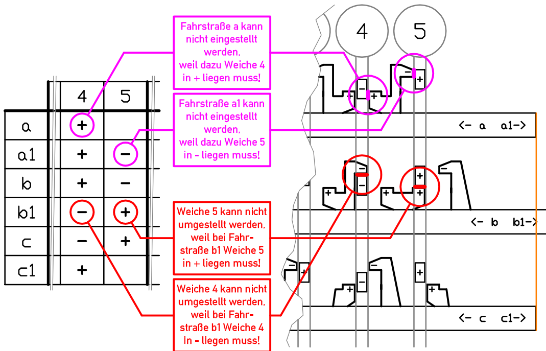
Beziehungen zwischen Verschlussplan und den Verschlussstücken. Fahrstraße b1 ist eingestellt.
