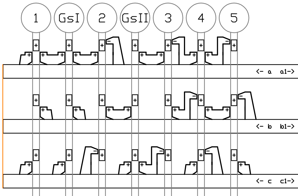
Grundstellung, keine Fahrstraße eingestellt
